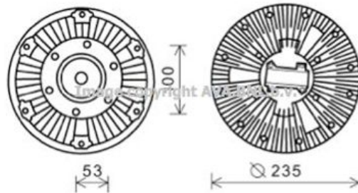
Fan clutch T114 C / 310 * 03/98-
